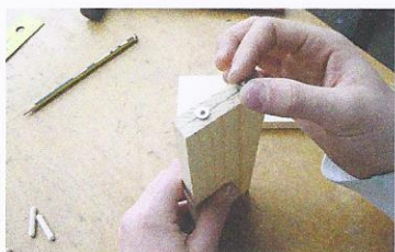
Vstavljanje prenosnih čepov
